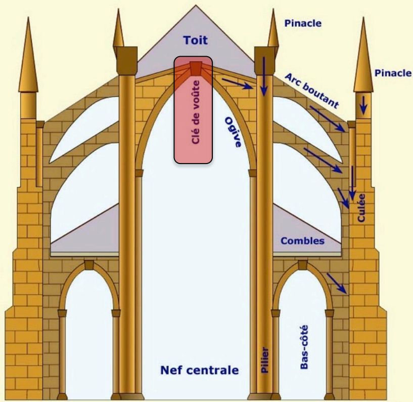
ART GOTHIQUE : Structure et poussées
