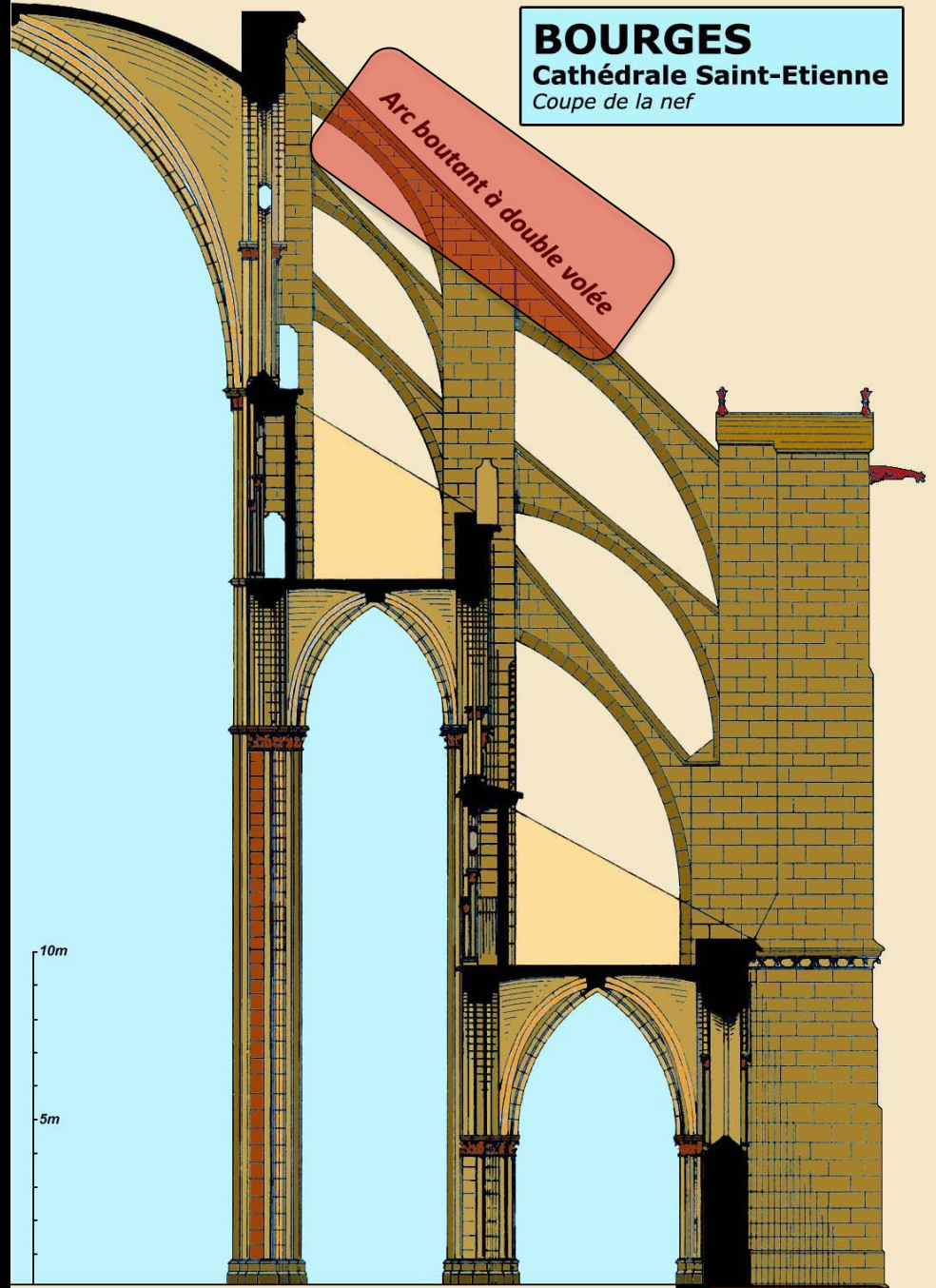
Nef centrale Premier collatéral Second collatéral Culée
